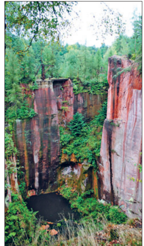
Auflässiger Steinbruch im Rochlitzer Porphyrtuff (Gleisbergbruch) auf dem Rochlitzer Berg.
