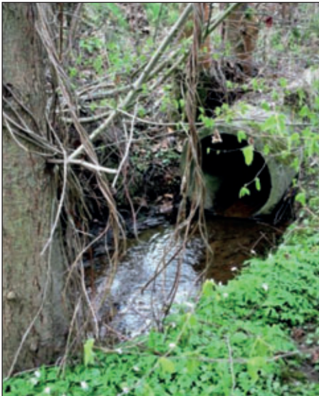
Unterführung der Bachwasserleitung an der Bundesstraße 175 /Foto: W&R Richter, Noßwitz 2020/
