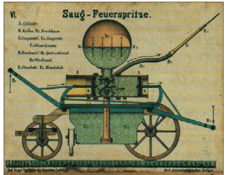
Plan einer Saug-Feuerspritze
