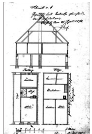
Bauzeichnung für den Bau des Schornsteines im Jahre 1876 und zugleich Darstellung der Räumlichkeiten des Hauses
